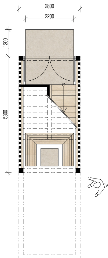
PŮDORYS NÁSTUPNÍHO PODLAŽÍ
